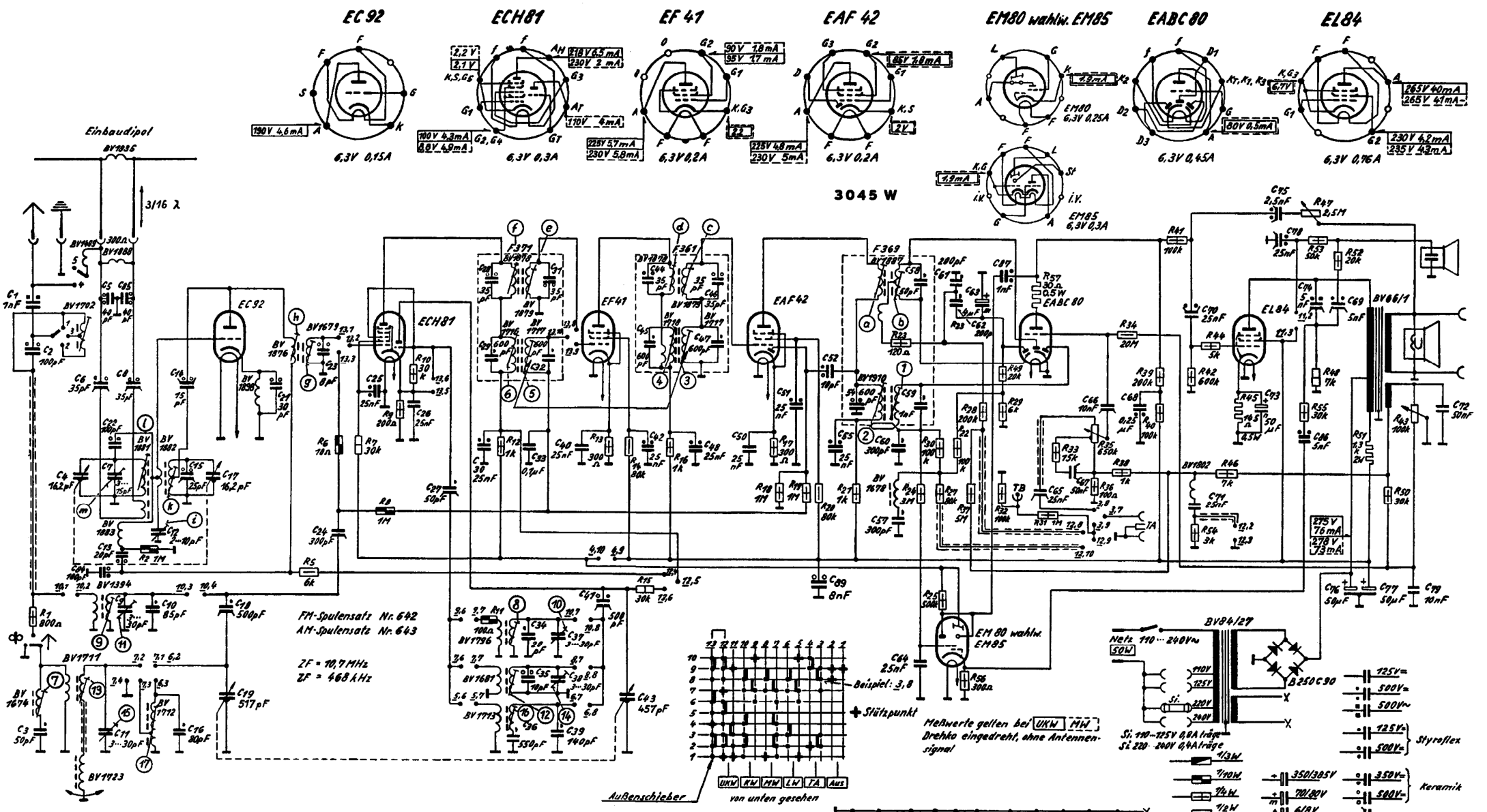
SCHALTPLAN 3045 W
